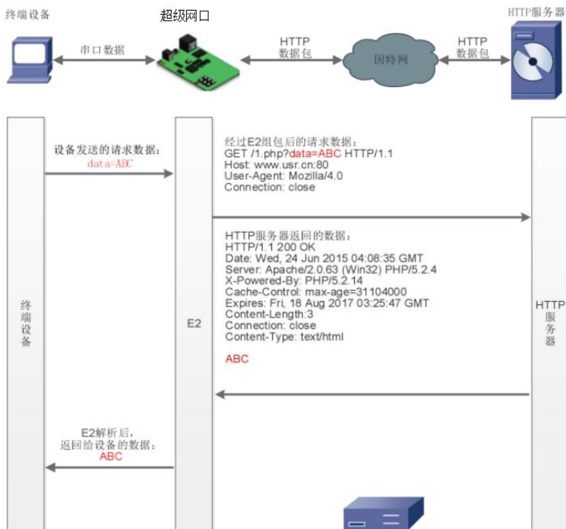
图 29 Httpd Client 模式说明
