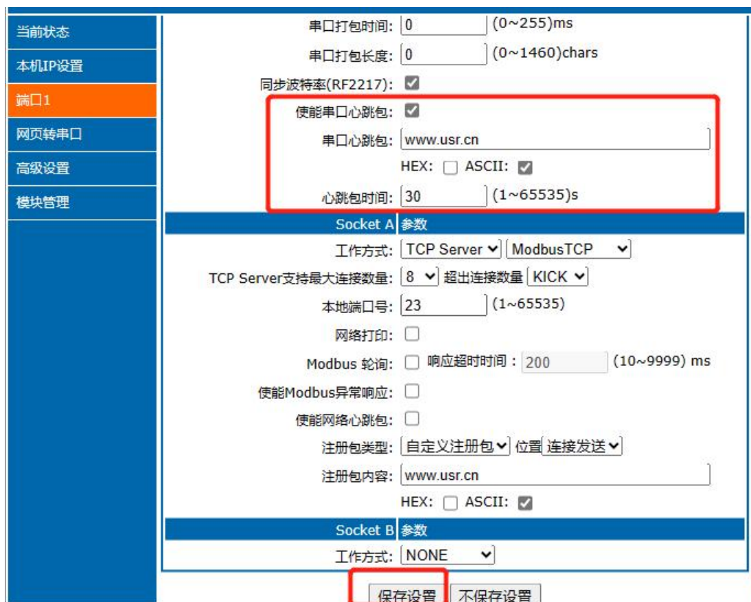
图 54 Modbus RTU 主动查询设置截图
