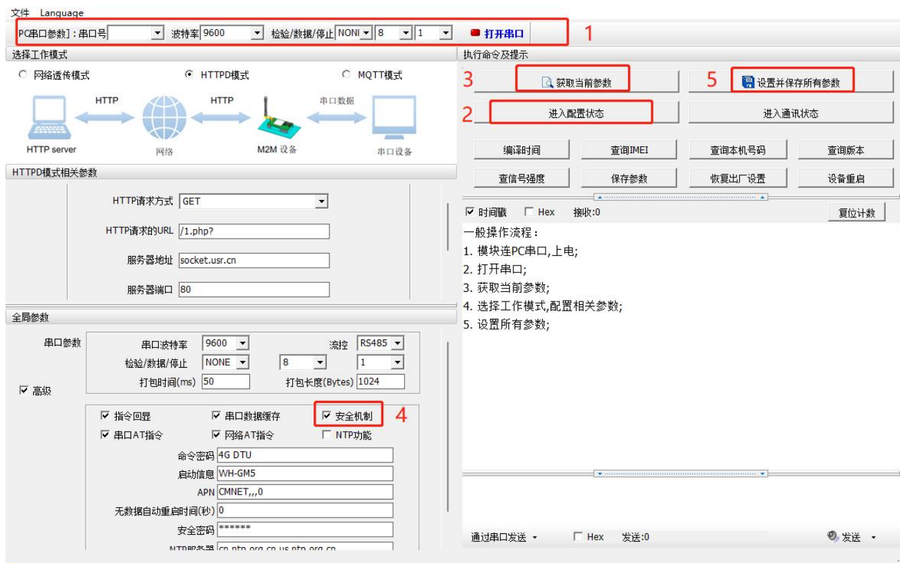
图 44. 设置软件示意图
