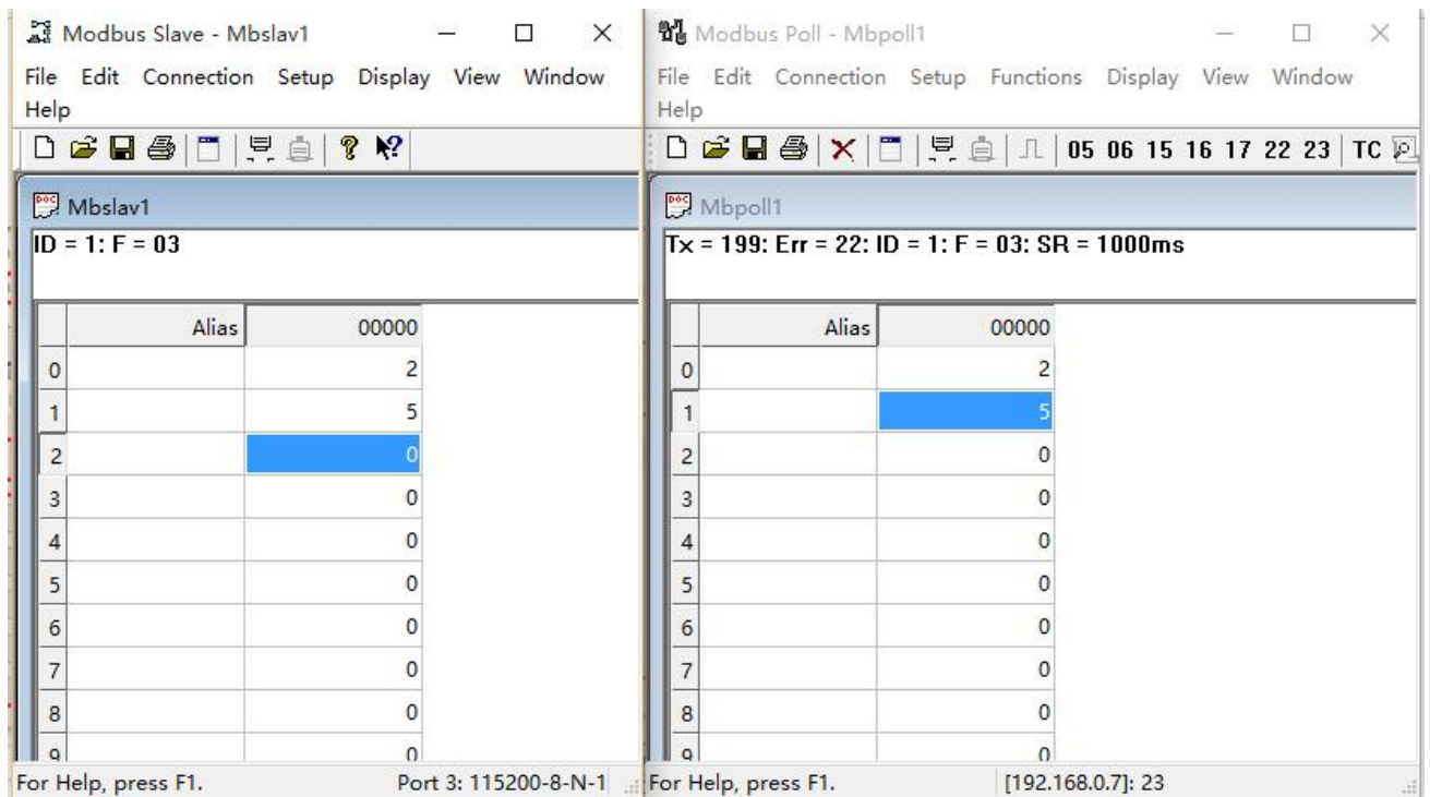
图 7. Modbus RTU 转 Modbus TCP 转换结果
