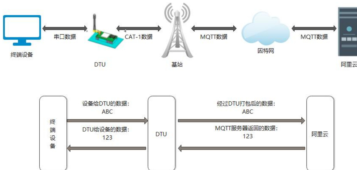
图 10. MQTT 模式
