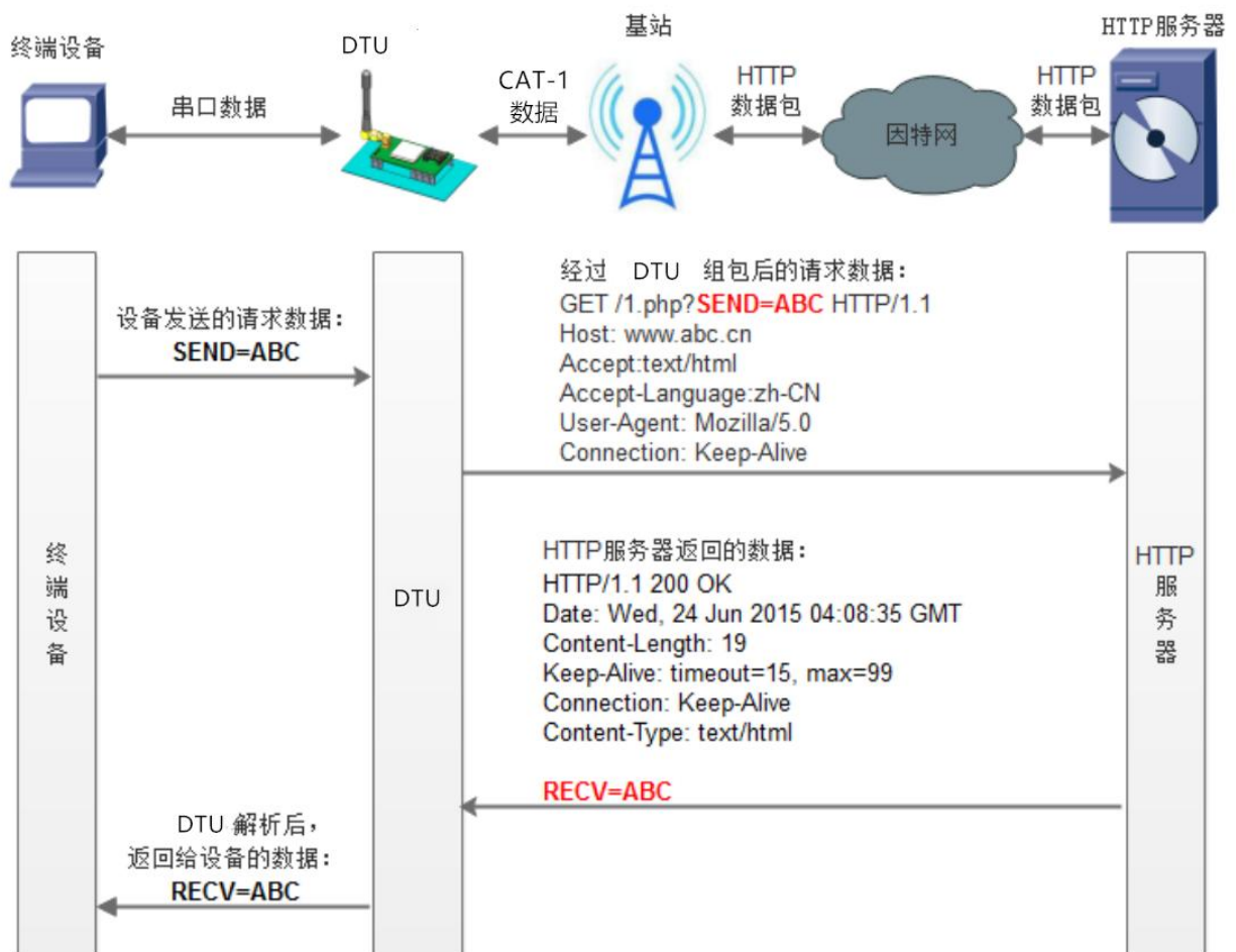
图 8. HTTPD Client 模式
