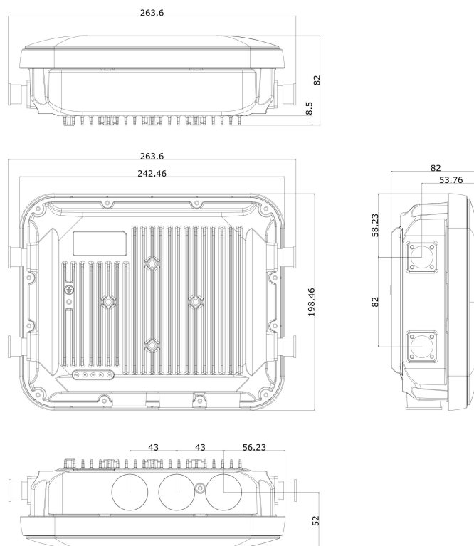
图 1 AP520X 尺寸图
